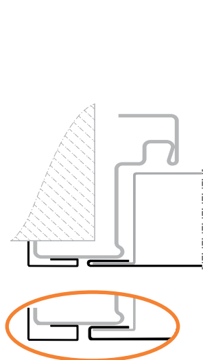
Eckzarge (Dünn-/Dickfalttür)
