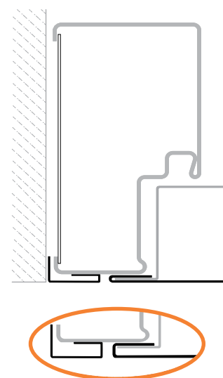
Blockzarge Typ 4.1 (Dünn-/Dickfalttür)
