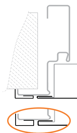
Umfassungszarge (Dünn-/Dickfalttür)
